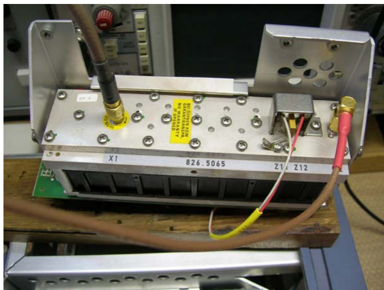
Abbildung 2: ausbaute Eichleitung im Test
