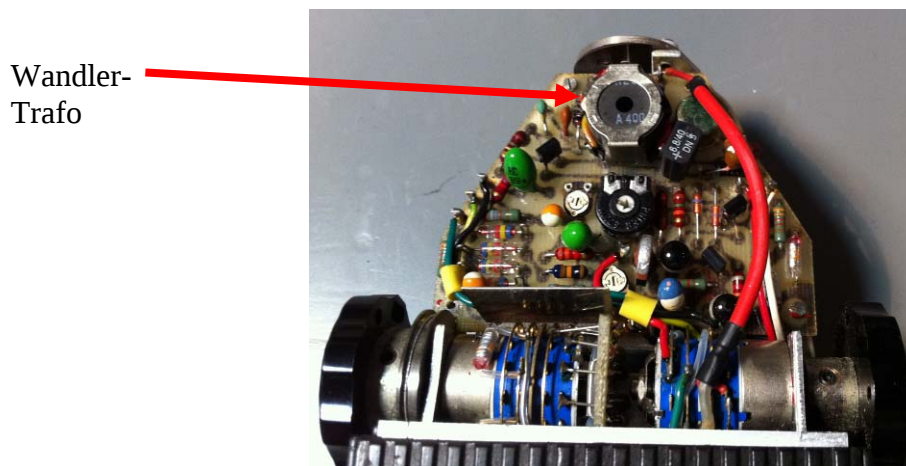
Abbildung 6: Schaltnetzteil(!) im 40 Jahre alten BK2205
